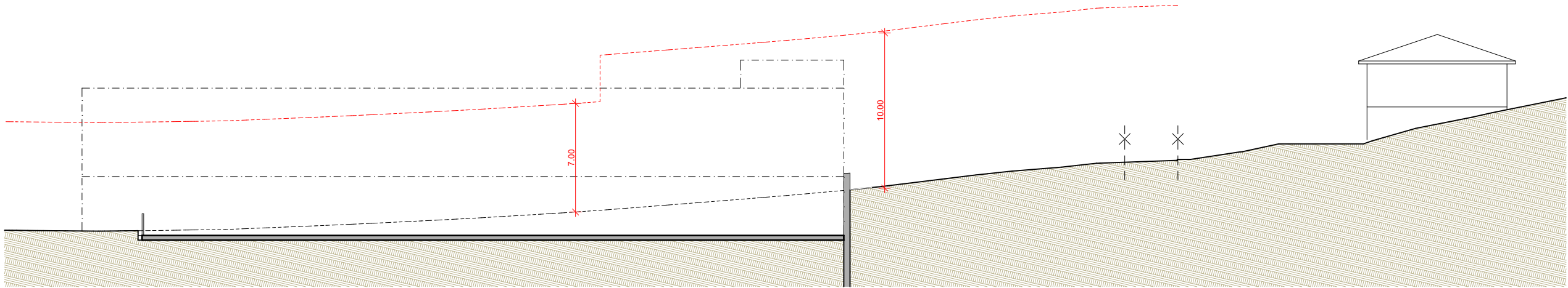
Schnitt
